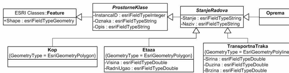
Figure 5 - Class diagram Tehnologija
